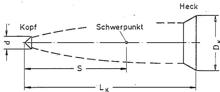
Prinzipskizze eines voll kavitierenden Körpers
